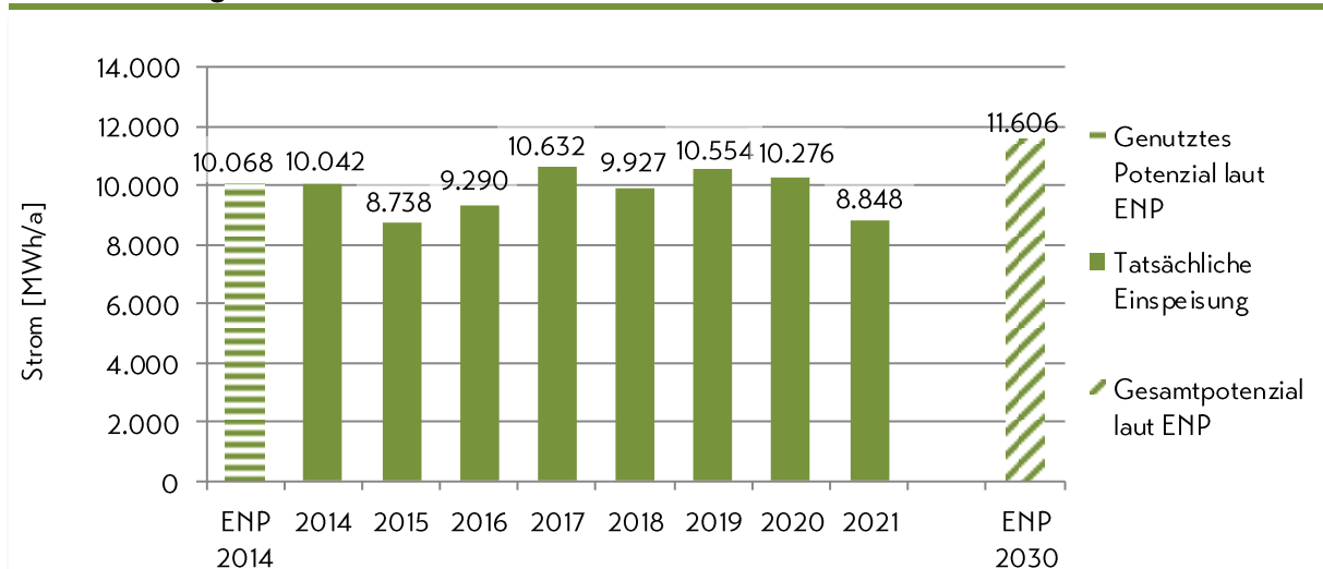
Abbildung 7: Stromerzeugung aus fester und flüssiger Biomasse (Netzeinspeisung) für den Zeitraum 2014 bis 2021 sowie das laut Energienutzungsplan im Jahr 2014 genutzte Potenzial und im Jahr 2030 mögliche Gesamtpotenzial
