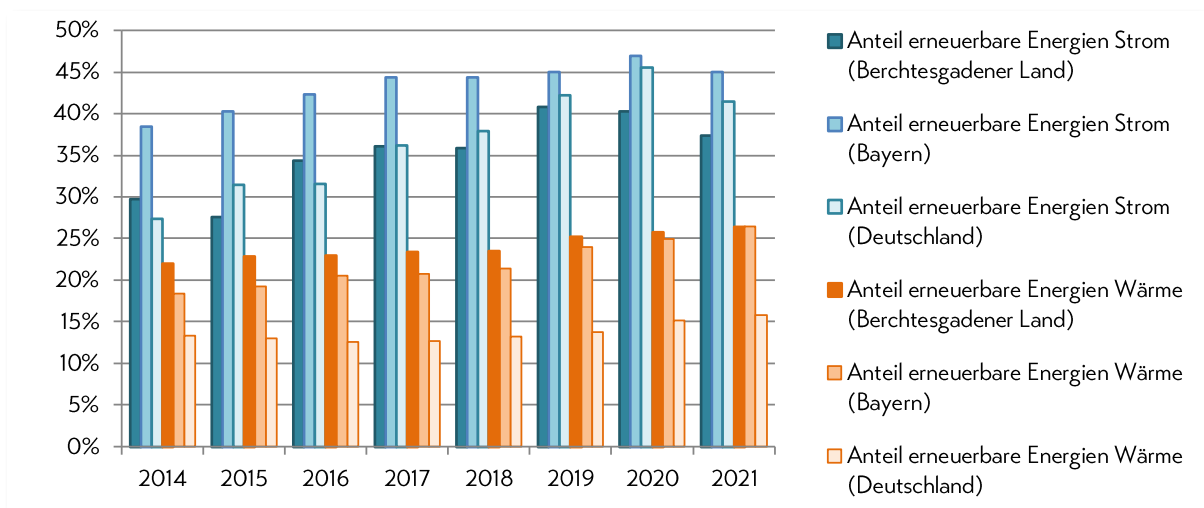
Abbildung 20: Anteile erneuerbarer Energien am Bruttostromverbrauch und an der Wärmebereitstellung (ohne Umweltwärme bzw. oberflächennahe Geothermie) für die Jahre 2014 bis 2021 im Vergleich für den Landkreis Berchtesgadener Land, Bayern und Deutschland (Quellen für überregionale Werte: StMWi, BMWK)
