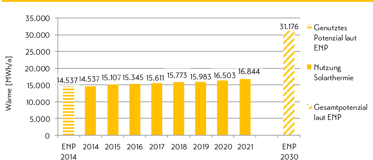
Abbildung 12: Wärmebereitstellung (Endenergie) aus Solarthermie für den Zeitraum 2014 bis 2021 sowie das laut Energienutzungsplan im Jahr 2014 genutzte Potenzial und gesamte erschließbare Potenzial bis 2030
