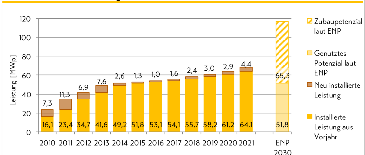
Abbildung 4: Installierte Photovoltaikleistung (kumuliert) im Landkreis Berchtesgadener Land für den Zeitraum 2010 bis 2021 sowie Ausbaupotenzial laut Energienutzungsplan (Quelle: Bundesnetzagentur, Marktstammdatenregister)
