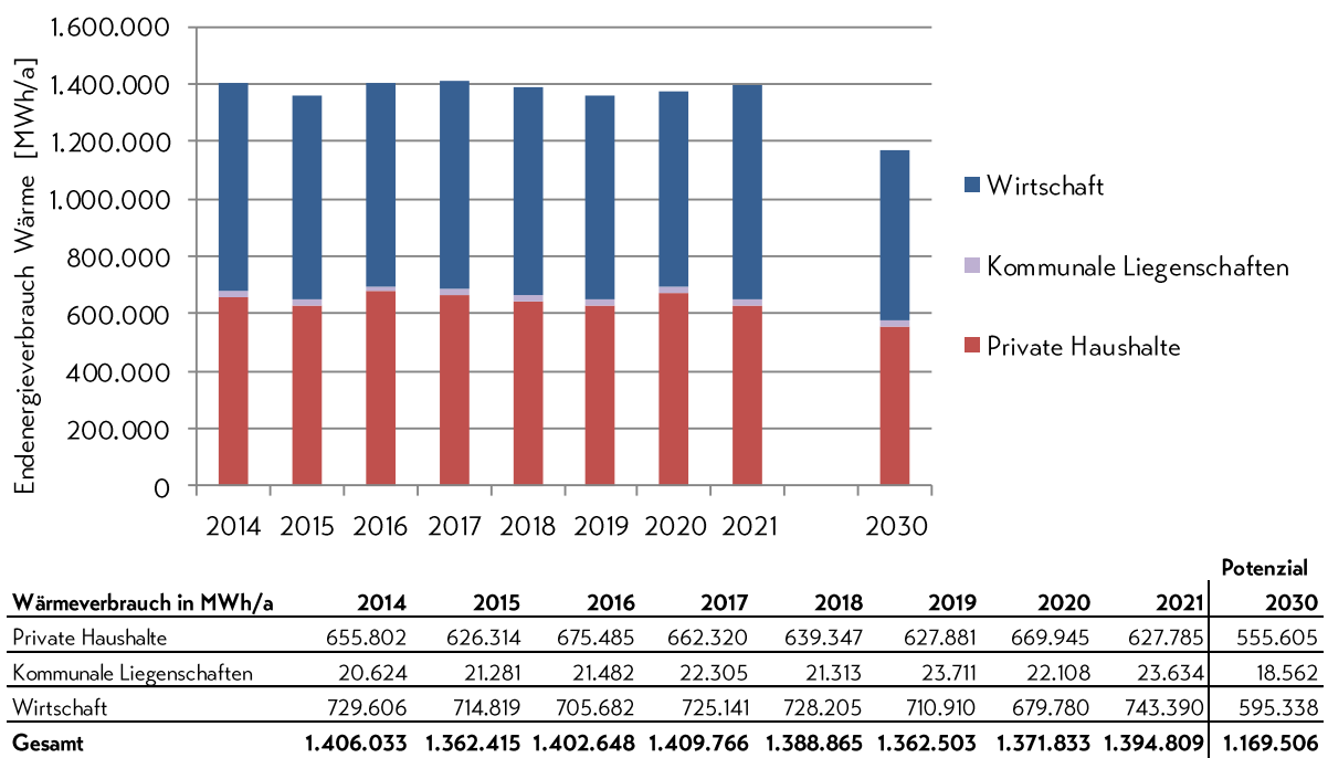
Abbildung 11: Wärmeverbrauch der einzelnen Verbrauchergruppen für den Zeitraum 2014 bis 2021 sowie das im Energienutzungsplan ausgewiesene Szenario für das Jahr 2030
