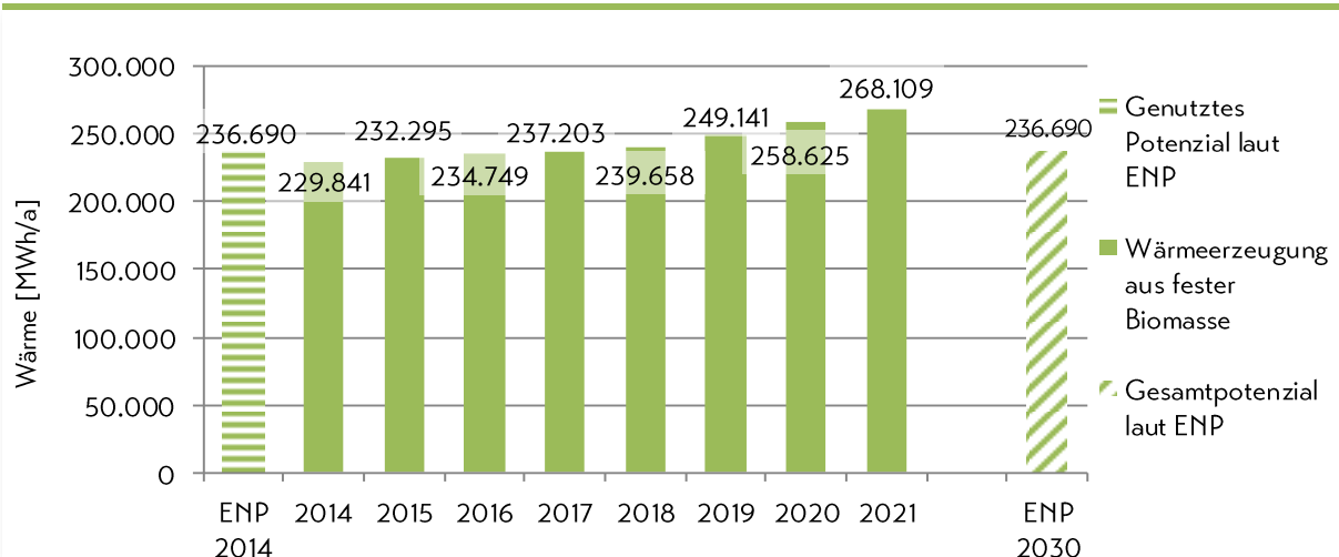
Abbildung 13: Wärmebereitstellung (Endenergie) aus fester Biomasse für den Zeitraum 2014 bis 2021 sowie das laut Energienutzungsplan im Jahr 2014 genutzte Potenzial
