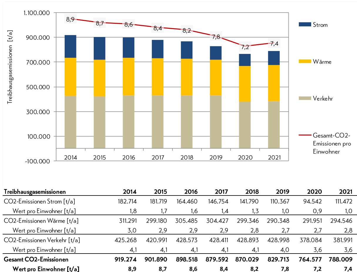
Abbildung 29: Treibhausgasemissionen unterteilt nach Sektoren für den Zeitraum 2014 bis 2021. Angabe in Tonnen-CO 2 -Äquivalente.
