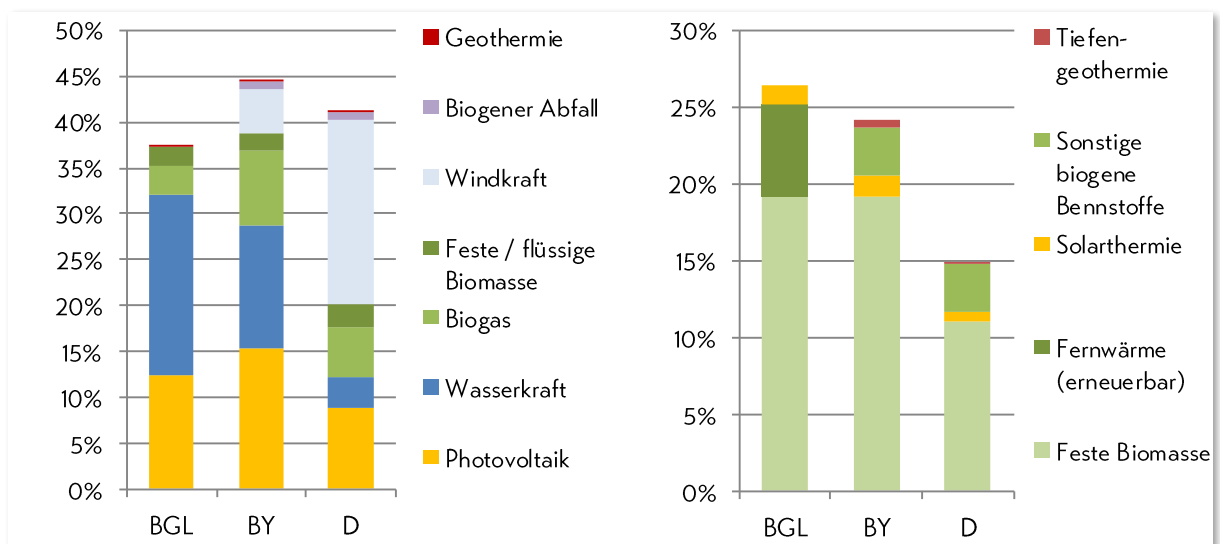
Abbildung 21: Anteile erneuerbarer Energieträger am Bruttostromverbrauch (links) sowie an der Wärmebereitstellung für das Jahr 2021 im Landkreis Berchtesgadener Land sowie in Bayern und Deutschland (Quellen für überregionale Werte: StMWi, UBA, BMWK)
