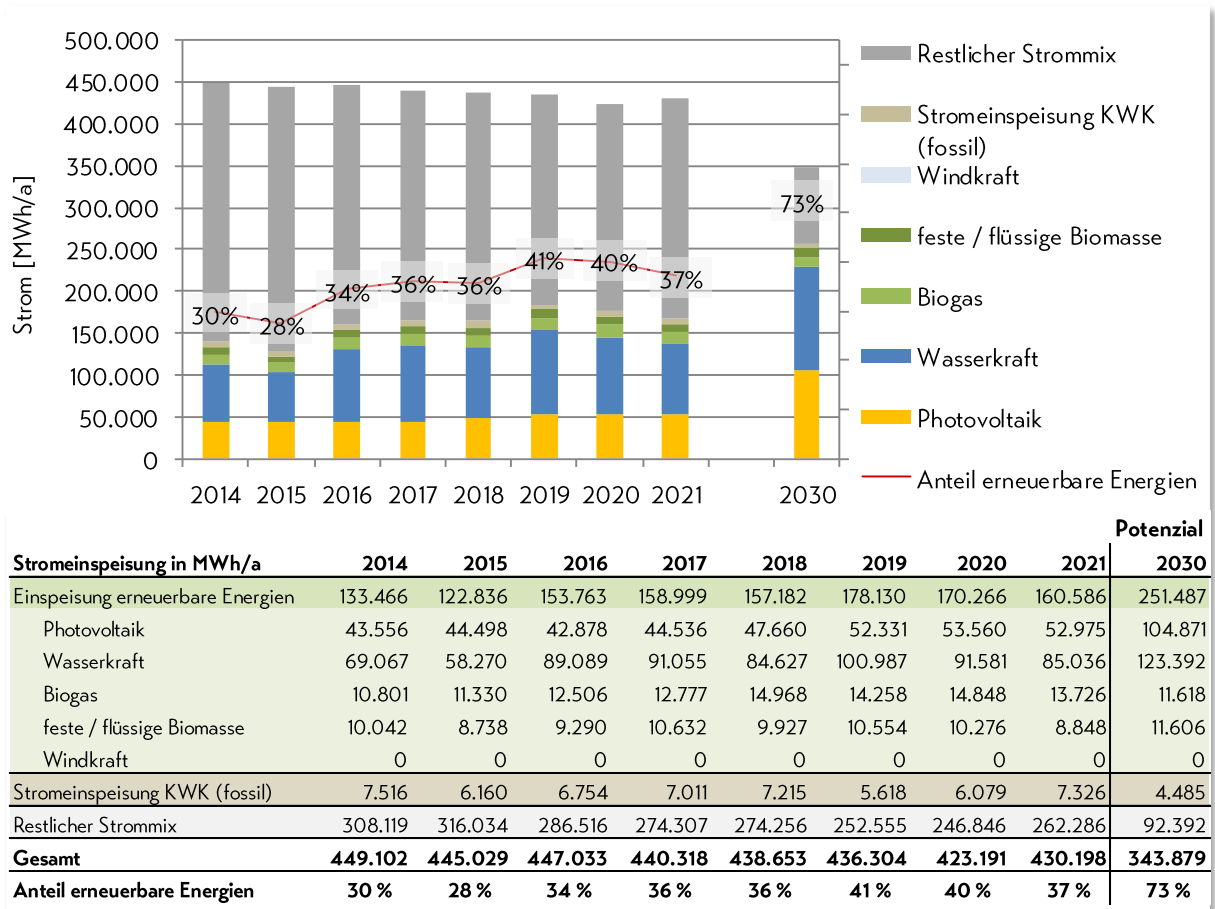
Abbildung 9: Strombezug und Einspeisung erneuerbarer Energien und KWK für den Zeitraum 2014 bis 2021 sowie das im Energienutzungsplan ausgewiesene Szenario für das Jahr 2030
