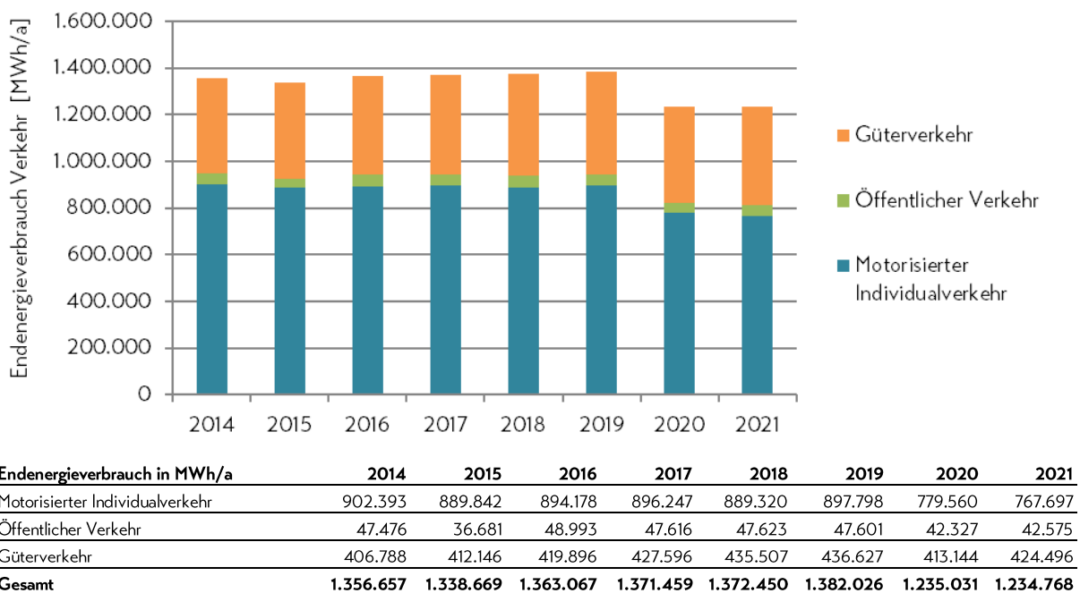
Abbildung 23: Endenergieverbrauch der einzelnen Verbrauchergruppen für den Zeitraum 2014 bis 2021 im Sektor Verkehr
