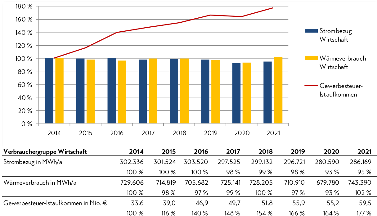
Abbildung 28: Endenergieverbrauch der Verbrauchergruppe Wirtschaft in den Sektoren Strom und Wärme sowie das Gewerbesteuer-Istaufkommen im Landkreis Berchtesgadener Land als Indikator für die Wirtschaftsleistung
