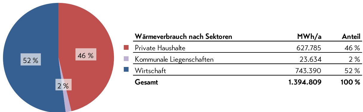
Abbildung 10: Wärmeverbrauch der einzelnen Verbrauchergruppen im Jahr 2021
