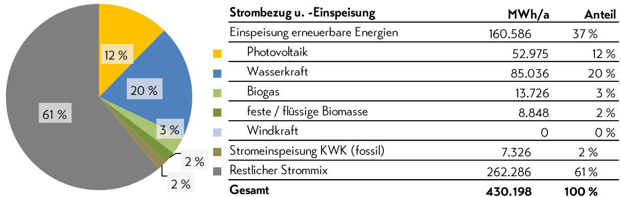
Abbildung 8: Strombezug und Einspeisung erneuerbarer Energien und KWK im Jahr 2021
