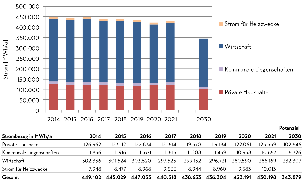
Abbildung 2: Strombezug der einzelnen Verbrauchergruppen für den Zeitraum 2014 bis 2021 sowie das im Energienutzungsplan ausgewiesene Szenario für das Jahr 2030.
