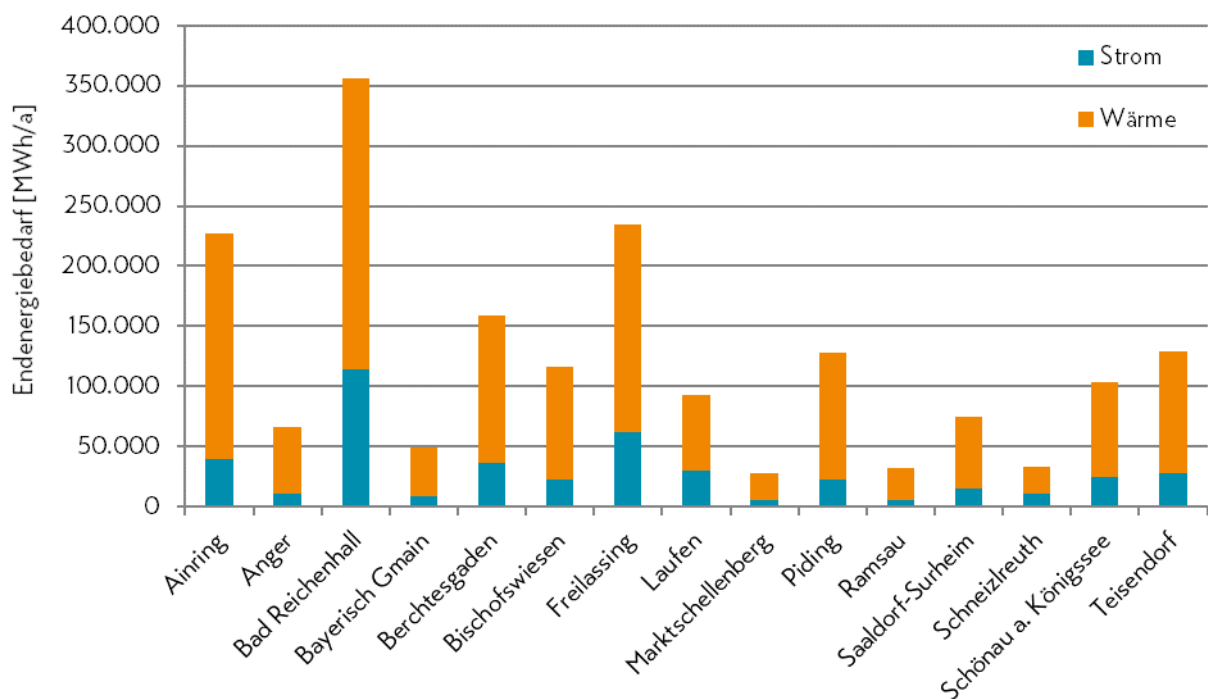
Abbildung 18: Endenergiebedarf für Strom und Wärme pro Kommune (2021)
