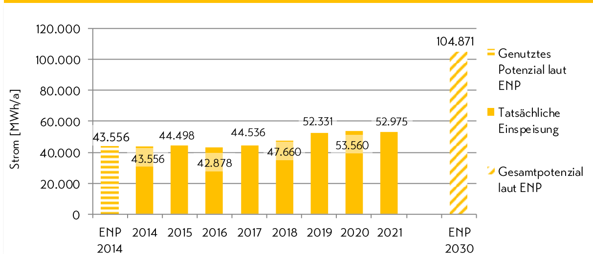
Abbildung 3: Stromerzeugung aus Photovoltaik (Netzeinspeisung) für den Zeitraum 2014 bis 2021 sowie das laut Energienutzungsplan im Jahr 2014 genutzte Potenzial und im Jahr 2030 mögliche Gesamtpotenzial
