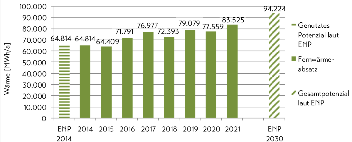
Abbildung 14: Fernwärmeabsatz auf Basis erneuerbarer Energien für den Zeitraum 2014 bis 2021 sowie das laut Energienutzungsplan im Jahr 2014 genutzte Potenzial und gesamte Potenzial bis 2030
