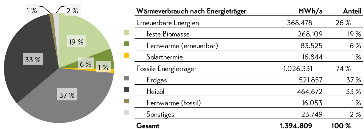
Abbildung 16: Wärmeverbrauch und Anteil der Energieträger in MWh im Jahr 2021
